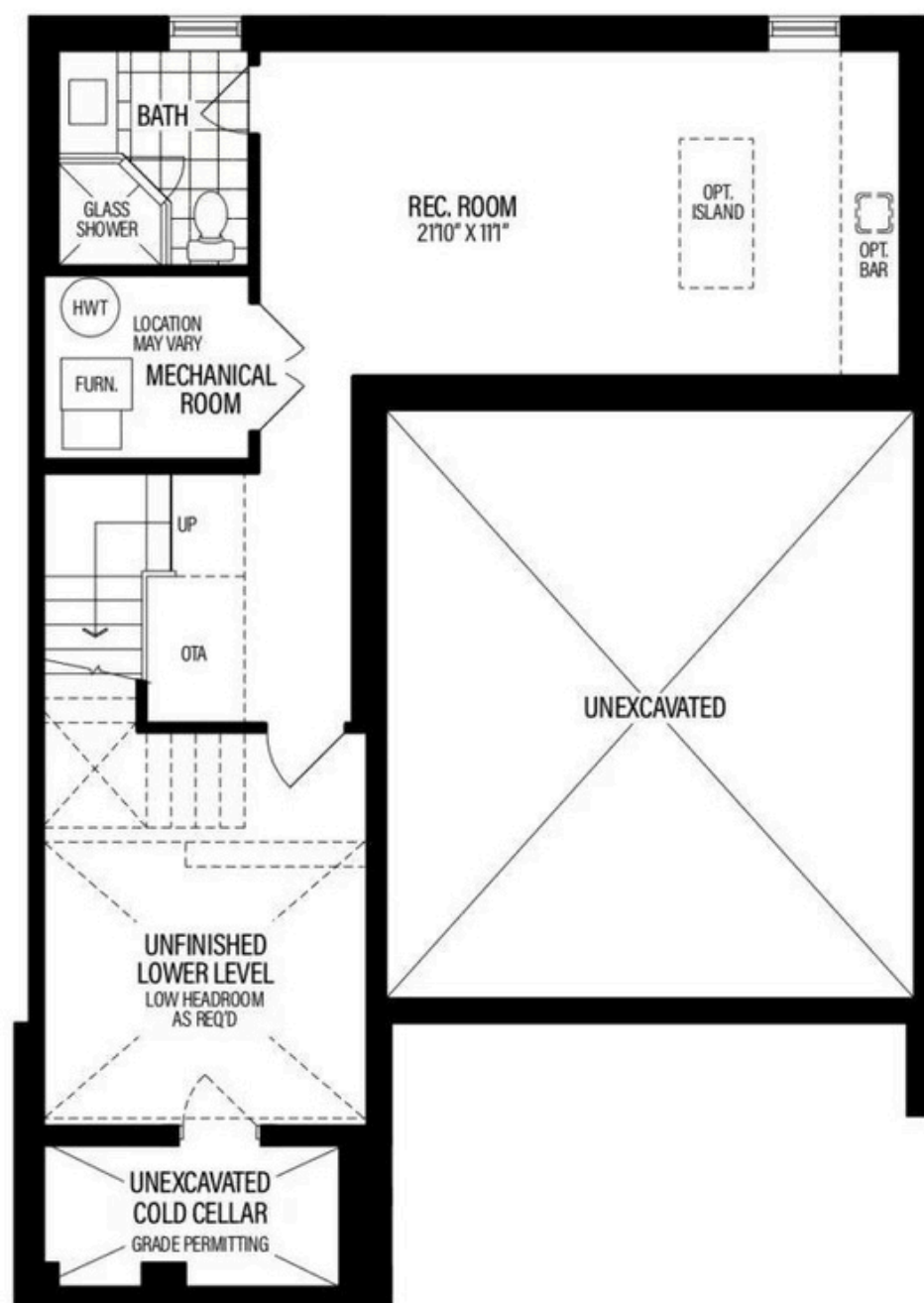
Lower Level ELEV 'A' & ELEV 'B'
