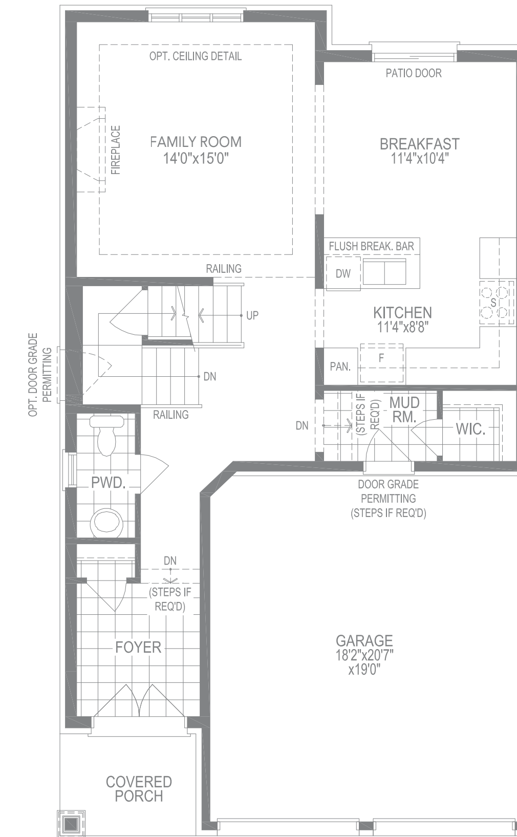
ELEV. A
