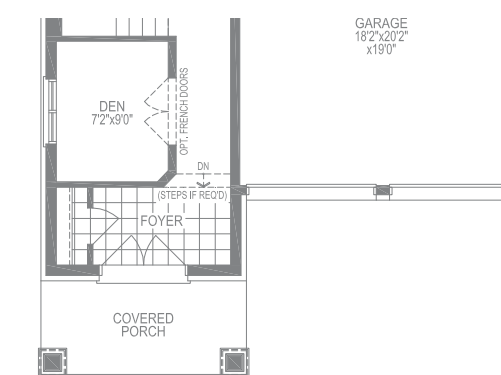
ELEV. B
