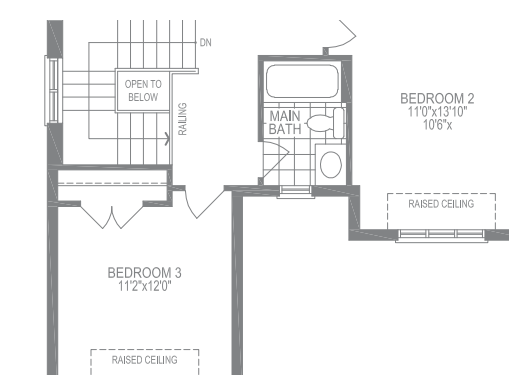
ELEV. B
