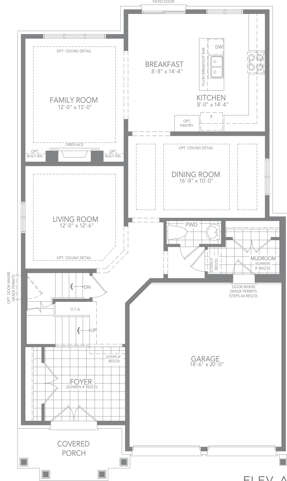
ELEV. A
