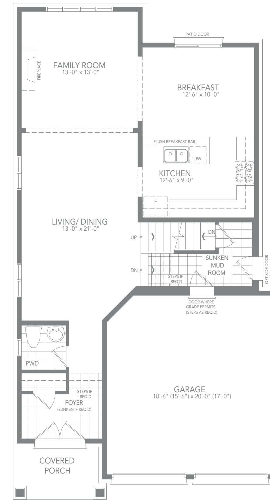
ELEV. A
