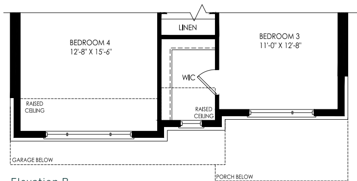
Elevation B
