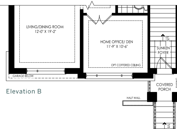
Elevation B
