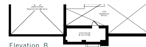
Elevation B
