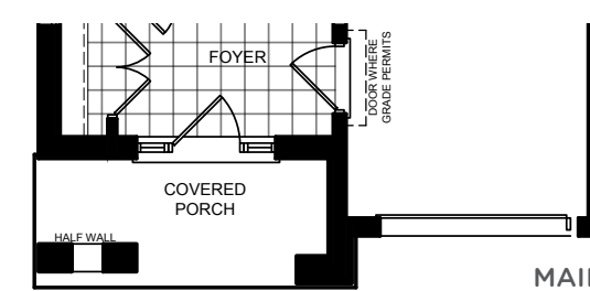
ELEV. C
