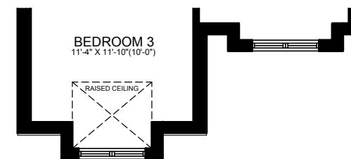
ELEV. B
