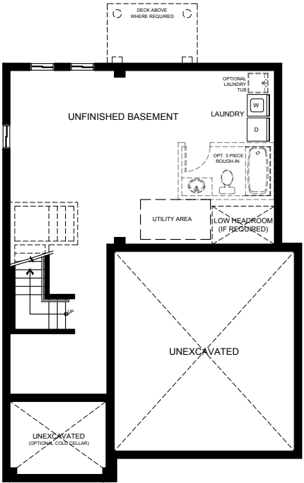
ELEV. A
