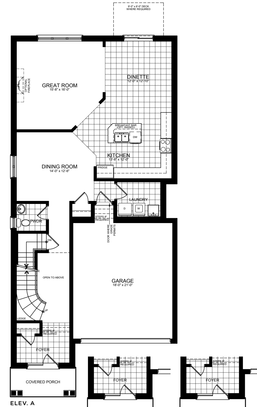
ELEV. A
