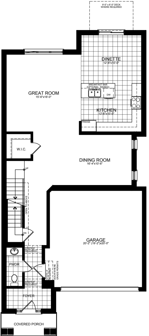
ELEV. A
