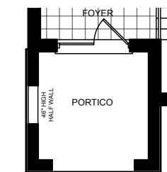
ELEV. B
