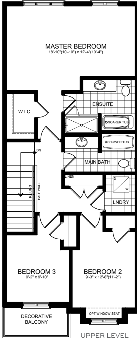
ELEV. A-2C
