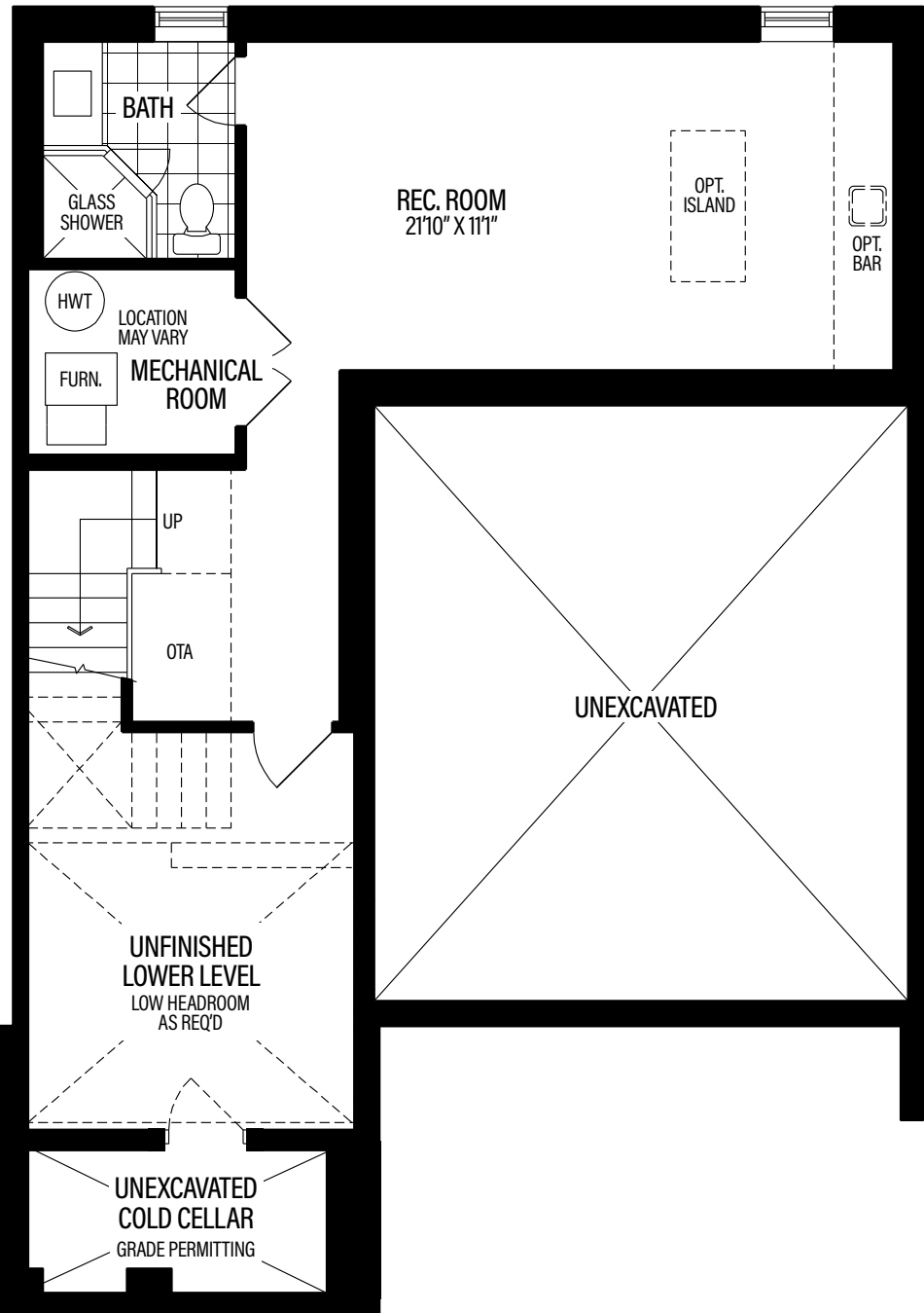
Lower level ELEV 'A' & ELEV 'B'
