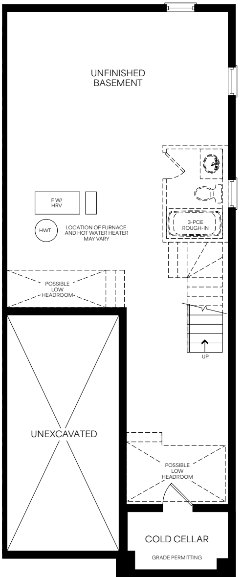
Basement Elevation A1 & A2
