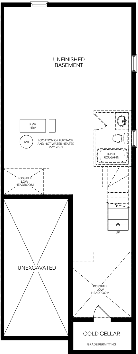
Basement Elevation A1 & A2
