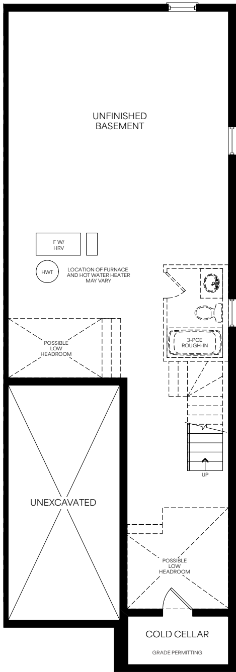
Basement Elevation A1 & A2
